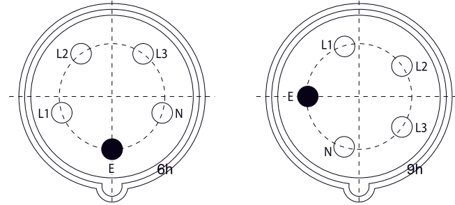
Prizin önden görünüşü
