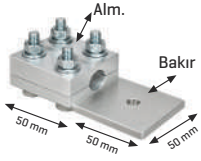
No: 3 Al-Cu Klemens
