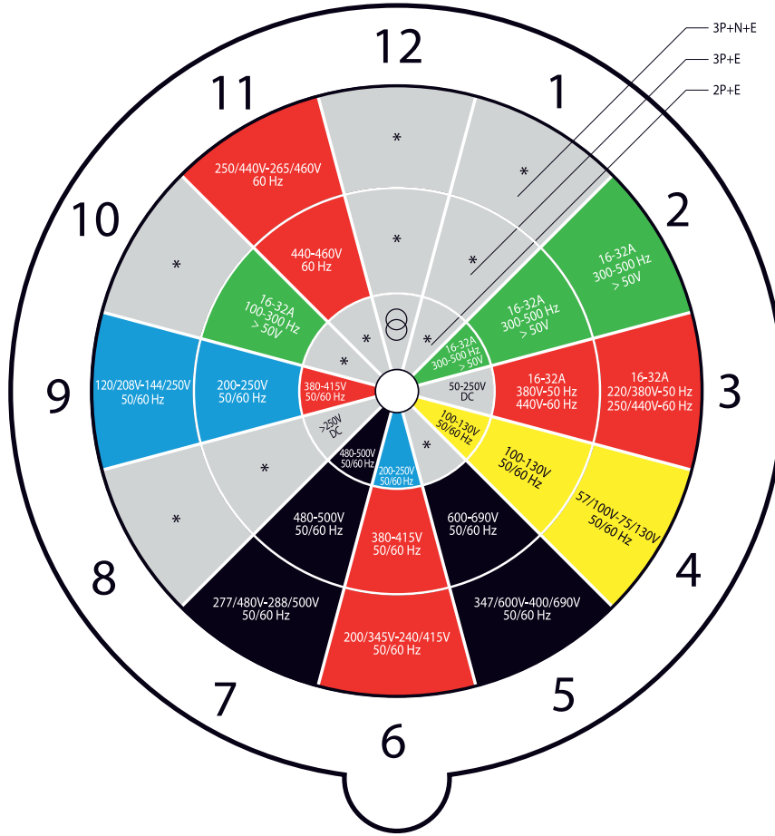
Prizin önden görünüşü
